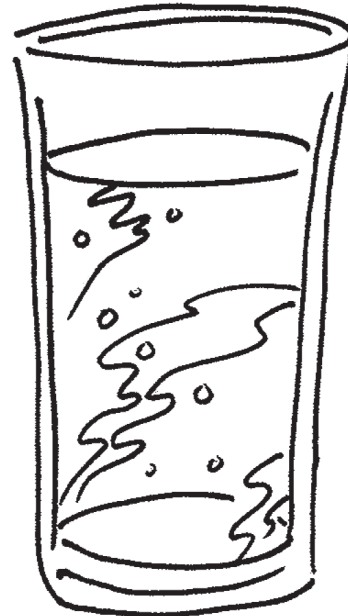
LIQUID (water)
